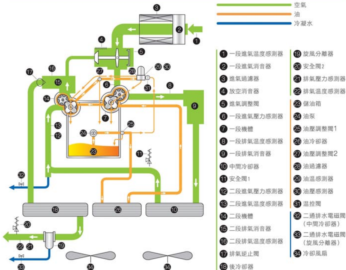
氣冷機-流程圖
